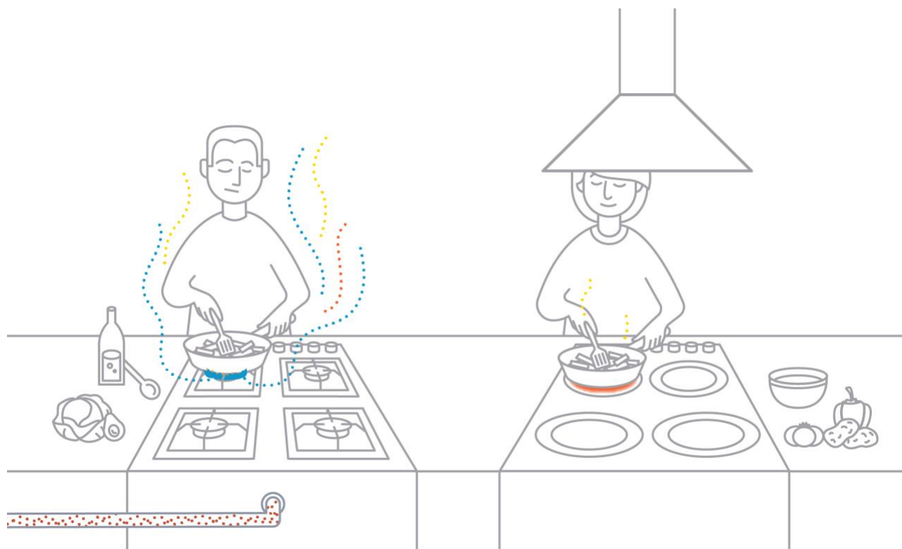
FIGURE 2. LE PASSAGE À LA CUISSON ÉLECTRIQUE RÉDUIT LES NIVEAUX DE POLLUTION DE L'AIR INTÉRIEUR CRÉÉE PAR LA BRÛLURE D'UN COMBUSTIBLE FOSSILE DANS LA CUISINE.
